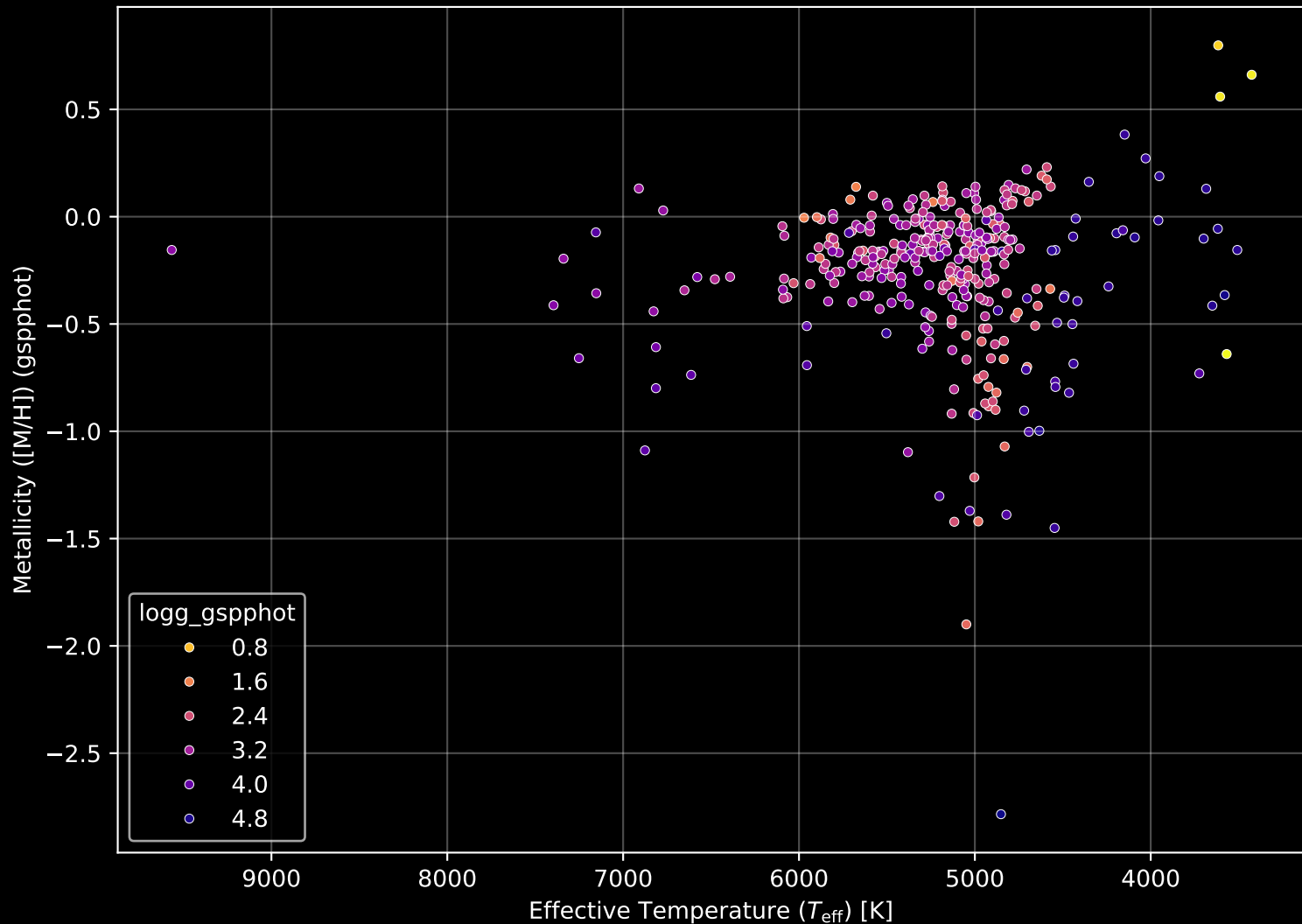
APOGEE DR17 Field: [000+17] Stellar Population Parameters (n= 354)
